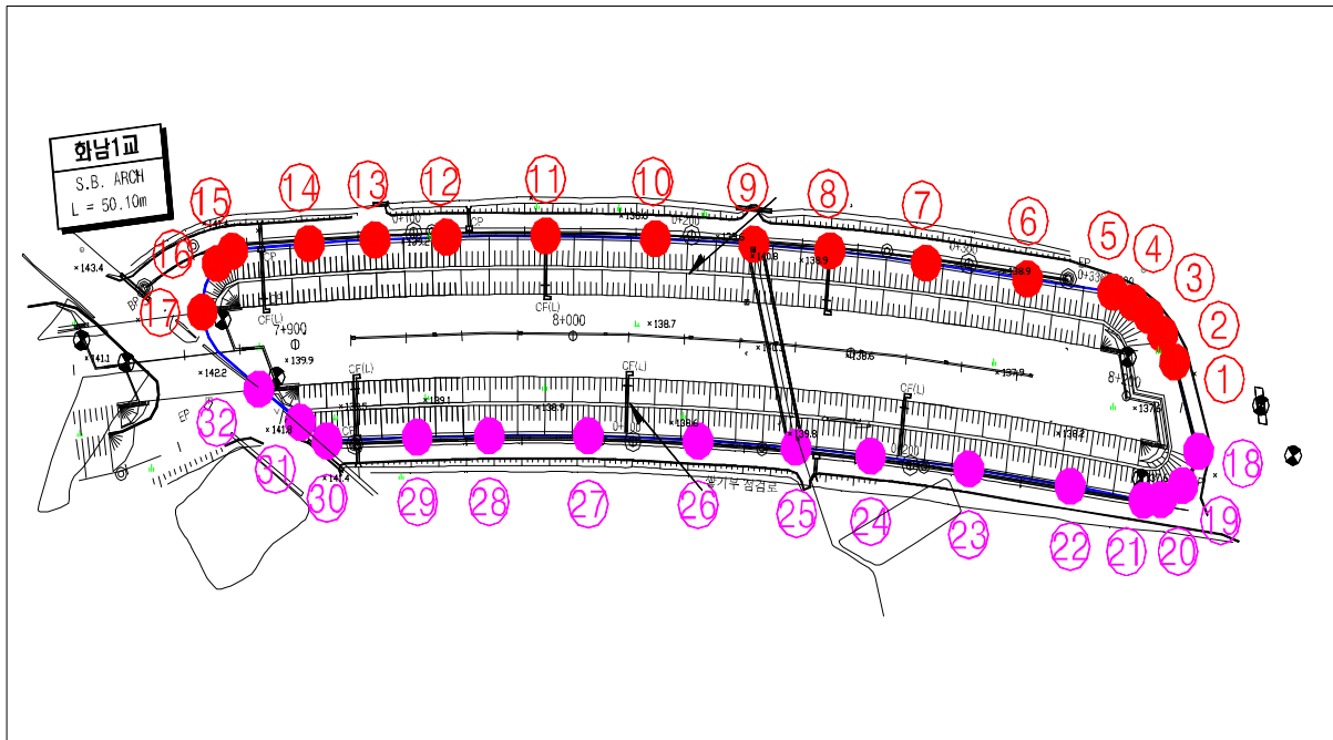
[ 선형측량 결과 ]
