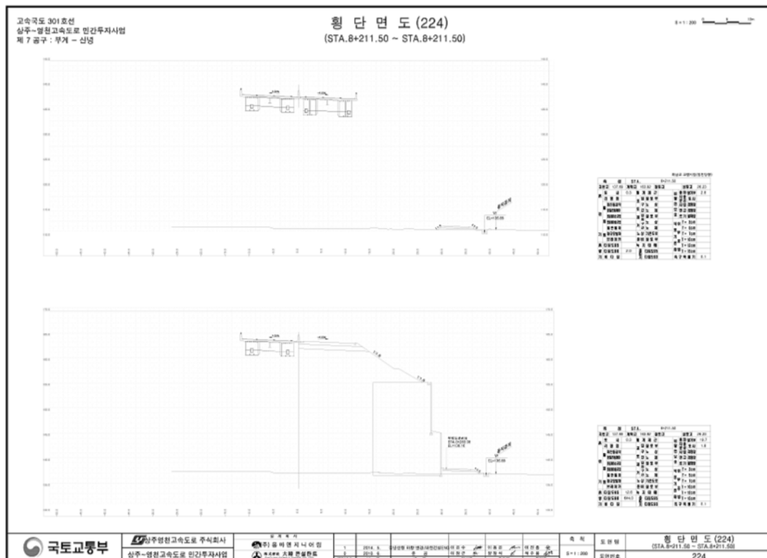
【그림 12.1.4】 단면도
