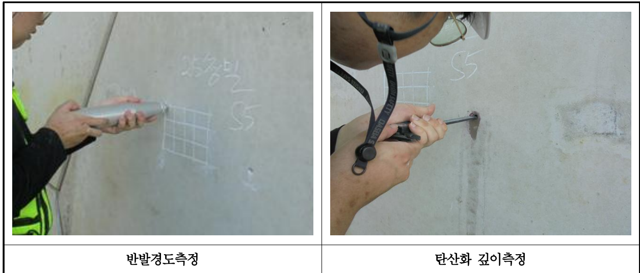
【사진 12.4.1】 재료시험 조사 전경
